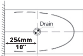
Gabarit d'installation
